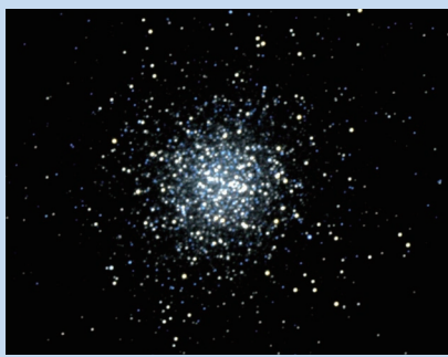
球状星団M13(天文館)
