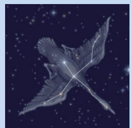
はくちょう座(イメージ)
